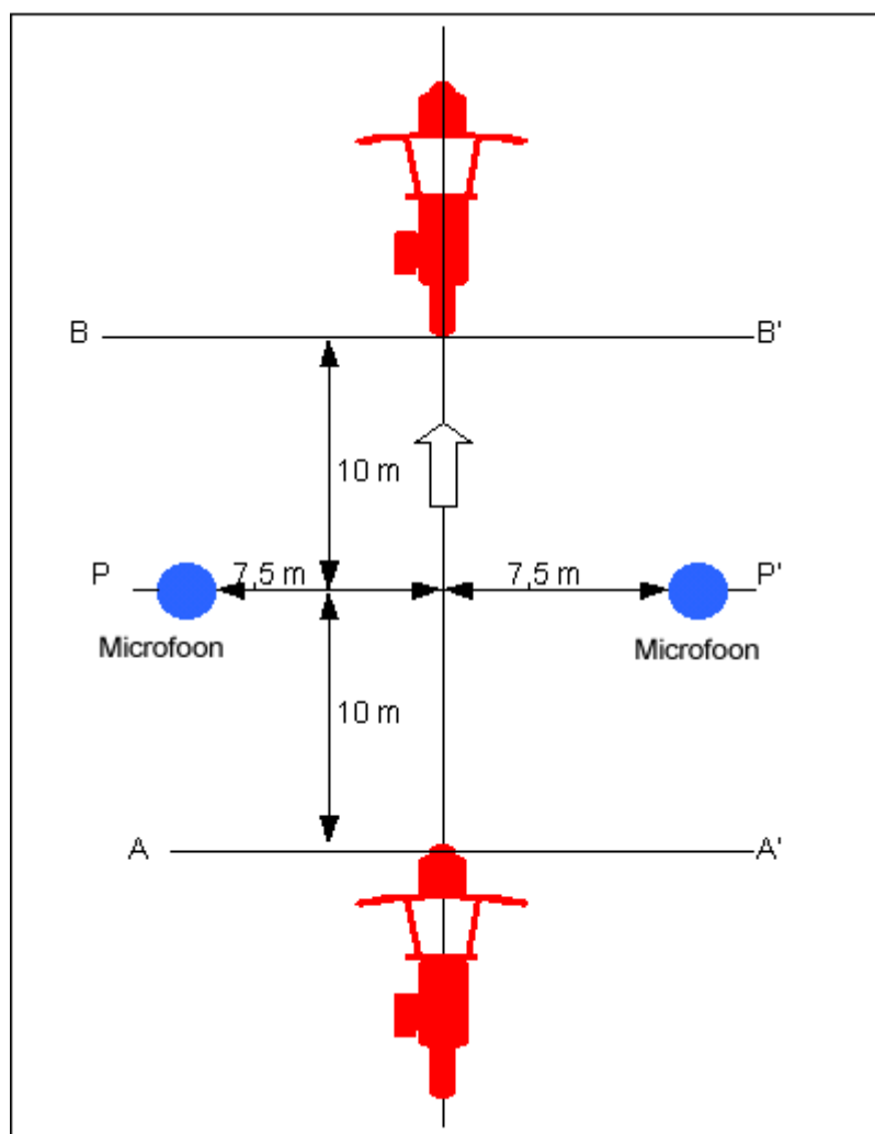
Proef bij stilstaande bromfiets
